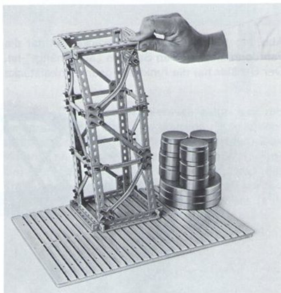
Abb. 26 Bei sehr starkem (mit dem Kraftmesser nicht mehr meßbarem) Druck auf eine Ecke können mehrere statische Funktionen einsichtig gemacht werden. Deutlich ist zu sehen, wie der Druck von rechts die obere Strebe biegt (Knickbelastung). Dasselbe geschieht an der unteren Strebe. Gegenkräfte erbringen entweder weitere Streben, die dann auf Zug belastet, den Druck abfangen oder Winkelträger, die sich nicht verformen. Der gesamte Turm ist bei dieser Belastung torsionsbeansprucht.
