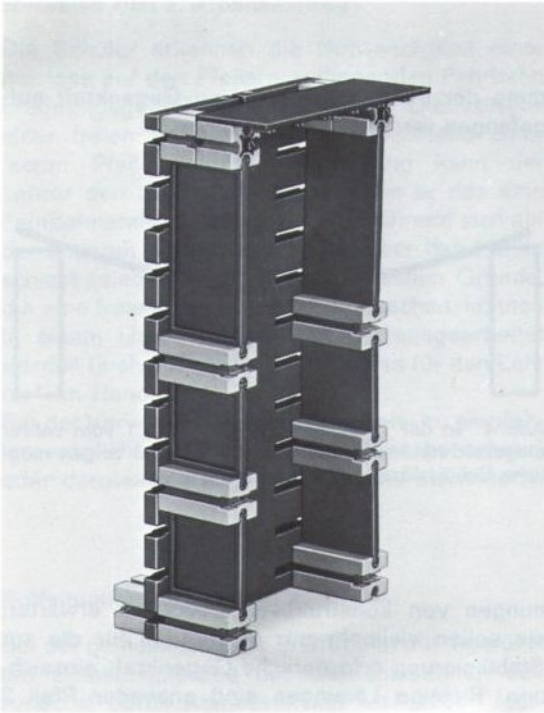
Abb. 1 In die große Grundplatte werden von unten her pro Seite je drei Bausteine 15 eingeschoben und mit Flachbausteinen 30 verbunden. Die Auflagefläche besteht aus einem Baustein 15 und einem Baustein 15 DV; dadurch kann, wie in den folgenden Beispielen zu sehen ist, die Bauplatte als „Andeutung“ zur Weiterführung der Fahrbahn durch einen Baustein 30 KL hochgehoben werden.
