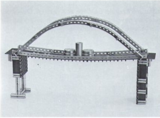
Abb. 11 Richtiges Anbringen der Bogenträger über den Auflagern bedeutet noch keine Stabilität der Fahrbahn. Es fehlt hier die Hauptsache: die „Verbindung“ zwischen tragendem Bogen und Fahrbahn in Form von Schnüren oder Streben.
