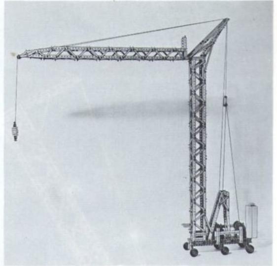
Abb. 36 Der Ausleger in der weitesten Auslage. Der Aufrichtebock am Ausleger ist hier ohne Funktion.
