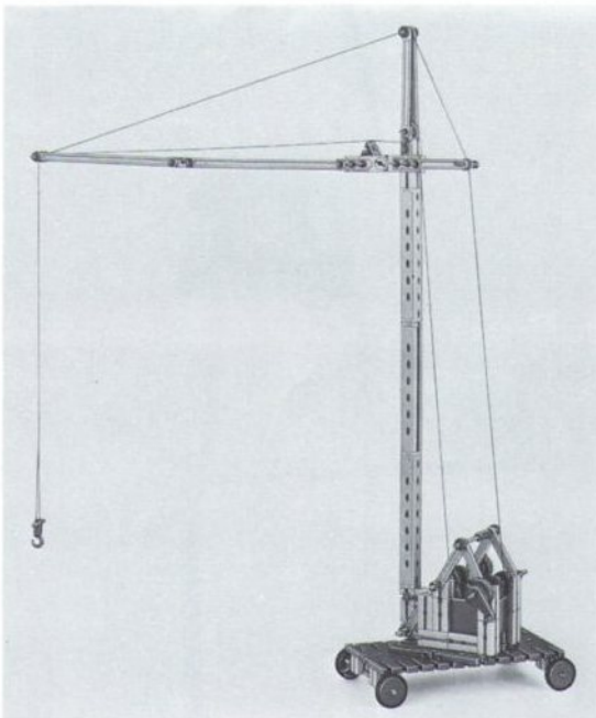
Abb. 29 Nach Arretierung des Turms in lotrechter Stellung und Lösen des Auslegers führt weiterer Seilzug zum Aufrichten des Nadelauslegers in die waagrechte Stellung (weiteste Auslage – kleinste Lastaufnahme). Erneuter Seilzug am Auslegereinziehwerk bewirkt ein Aufrichten des Auslegers in die steile Stellung (kleinste Auslage – größte Lastaufnahme).
