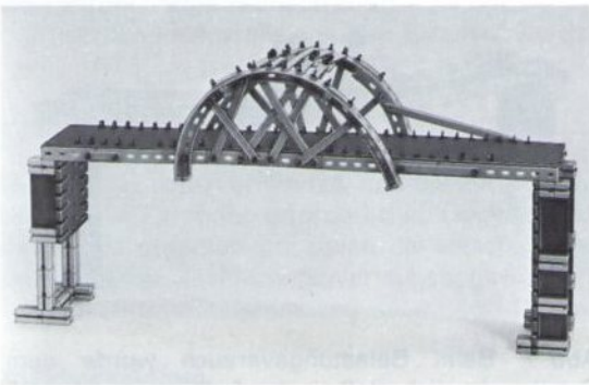
Abb. 9 Typisches Beispiel einer durch unreflektiertes „Vorwissen“ zustande gekommenen „Bogenbrücke“. Ohne Belastung erscheint die Lösung zunächst tauglich, weil die eingezogenen L-Winkelprofile als „Balken“ wirken.
