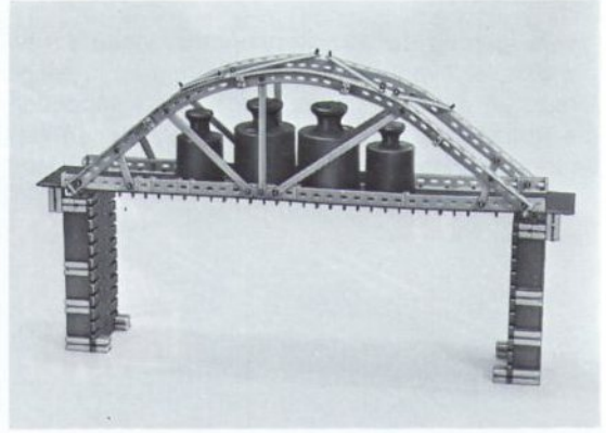
Abb. 12 Jetzt übernehmen die Streben einen Teil der Fahrbahnlast, „übergeben“ sie an die Bogenträger und diese „leiten“ sie auf die Auflagern ab. (Daß die Streben hier noch nicht symmetrisch angeordnet sind, und auch nur an einem Punkt der Fahrbahn angreifen, so daß sich besonders rechts noch Biegung zeigt, führte den Schüler zu einer gleichmäßigen über die ganze Fahrbahn verteilten Verstrebung.)
