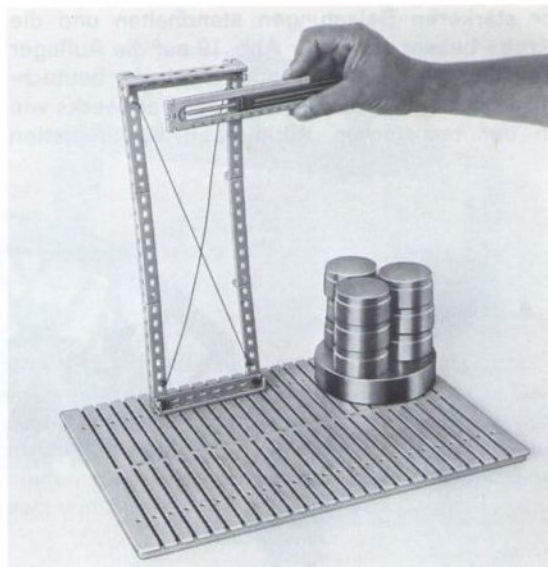
Abb. 24 Bereits die Diagonalverspannung mit Schnüren erbringt eine erhebliche Stabilisierung; jedoch ist hier nur in einer Ebene stabilisiert.
